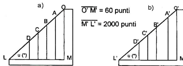
FIGURA 3. a) Se fijan intervalos de distancia iguales entre sí, midiendo el tiempo que el móvil tarda en recorrerlos(ver texto); b) Medir mediante múltiplos de tiempo los intervalos de distancia recorridos por el móvil(ver texto).
