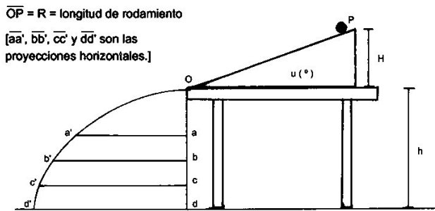
FIGURA 1. Reconstrucción del dispositivo experimental sugerido por Guidobaldo a Galileo
