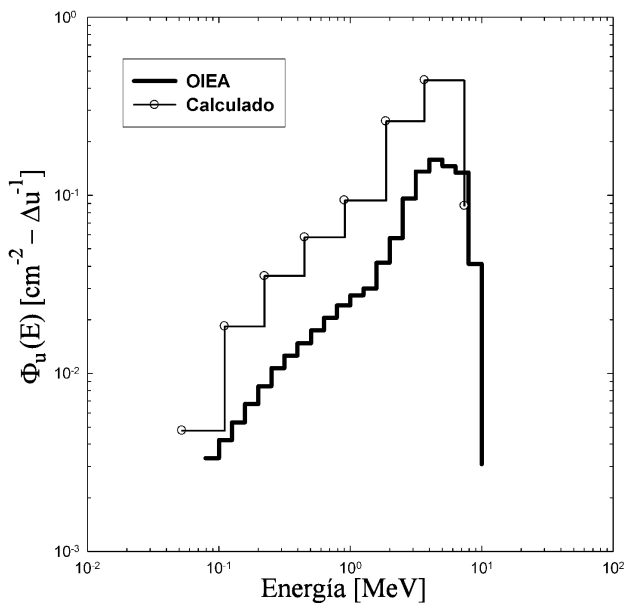
FIGURA 1. Espectro de los neutrones emitidos por la fuente de 241 AmBe.
