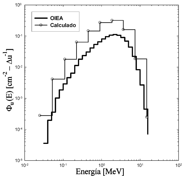
FIGURA 2. Espectro de los neutrones emitidos por la fuente de 252 Cf.
