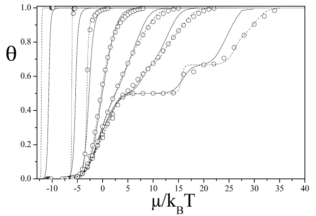
FIGURA 1. Isothermas de adsorción para dímeros alineados en dos dimensiones. De izq. a der.: \beta w = -4, -2, -1, 0, 1, 2, 4 . Líneas sólidas: solución de las ecs. cinéticas; rayas: solución de la gran función de partición; símbolos: simulación de Monte Carlo.
