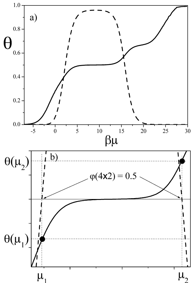
FIGURA 2. a) Representación esquemática del cálculo del diagrama de fase correspondiente a dímeros en dos dimensiones con interacciones repulsivas. b) Detalle del cálculo del diagrama de fase. Con línea sólida se grafica la isoterma de adsorción y con rayas la probabilidad de la configuración de la estructura ordenada c(4 \times 2) .
