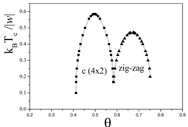
FIGURA 3. Diagrama de fase para dímeros alineados en un cluster con interacción lateral a primeros vecinos repulsiva obtenido mediante las ecuaciones cinéticas.
