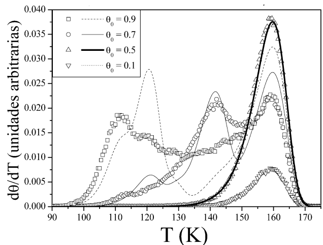
FIGURA 4. DTP inmóviles para interacción lateral repulsiva w = 0.5 kcal/mol y distintos cubrimientos iniciales \theta_0 . Con líneas: solución de las ecs. cinéticas; símbolos: simulación de Monte Carlo.
